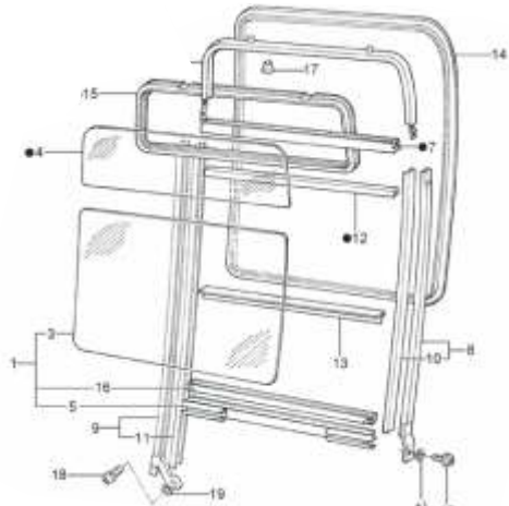
Vidro Janela
